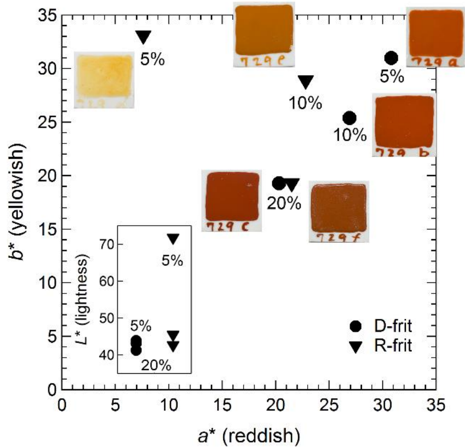
図6 D-フリットとR-フリットから作製した赤絵試片の外観写真と L^* , a^* , b^* 値。 図中の数字はヘマタイト濃度を示す。 Reprinted with permission from ref 19. Copyright 2018 John Wiley & Sons.
