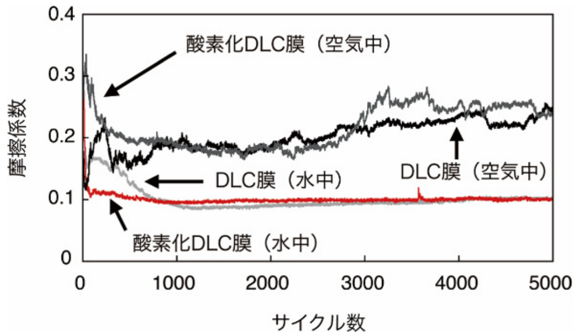
図20 空气中および水中における酸素官能基化反応処理前後のDLC膜の摩擦試験 (カラー版は当協会 HP に掲載)
