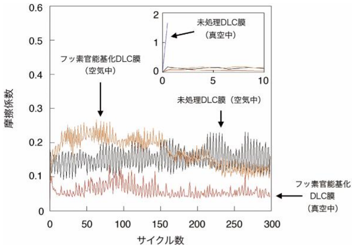
図17 空气中および真空中における 未処理およびフッ素官能基化 処理 DLC 膜の摩擦特性 (カラー版は当協会 HP に掲載)
