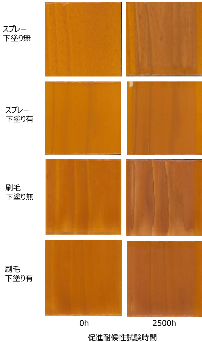
図3 CNF添加下塗り用塗料を異なる塗装方法で塗装した試験片の外観
