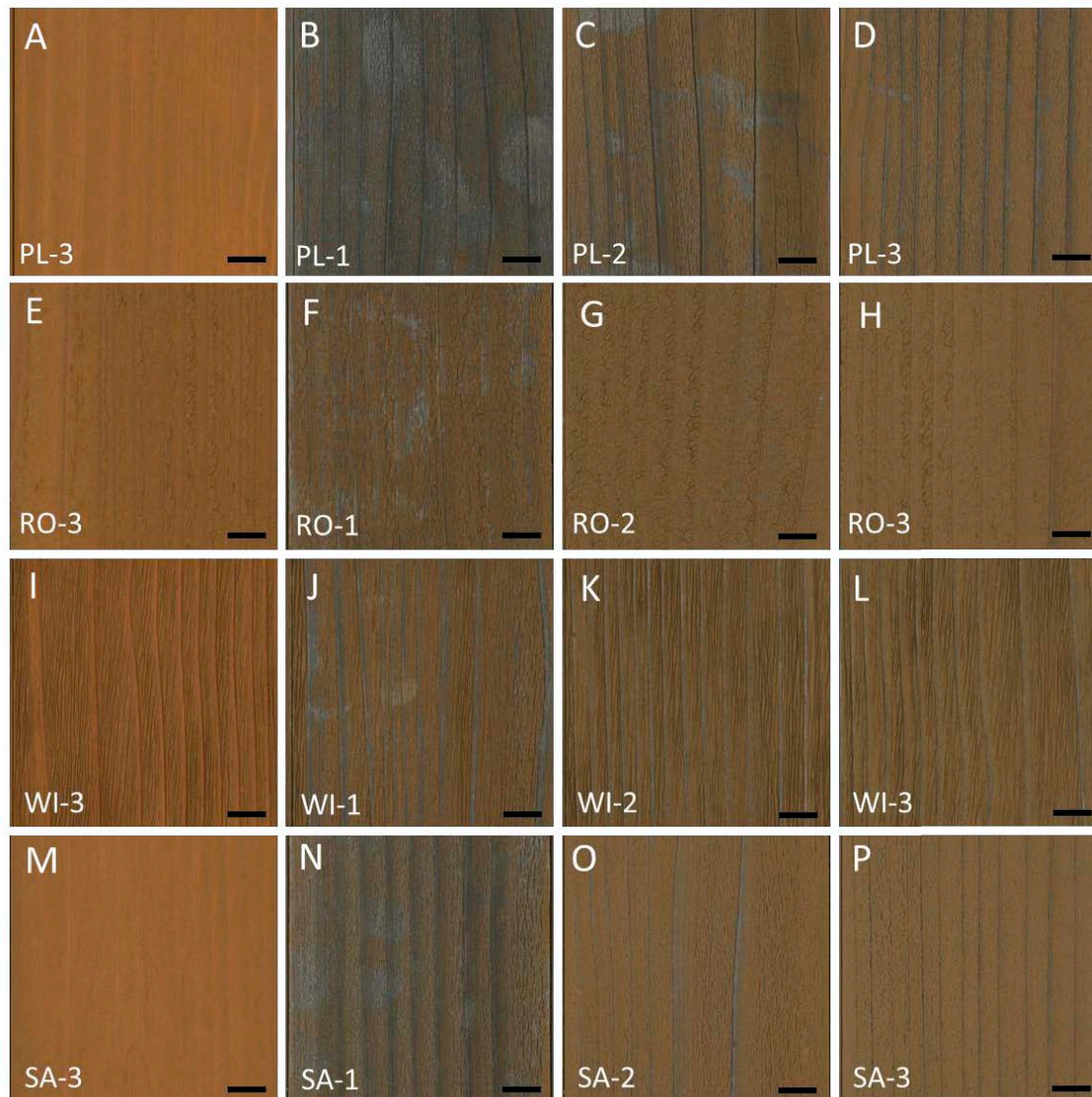
図6 暴露前および屋外暴露7年経過後の塗装面の外観 記号は表1を参照、A,E,I,M: 暴露前、B-D, F-H, J-L, N-P: 暴露7年後、 bar: 10 mm
