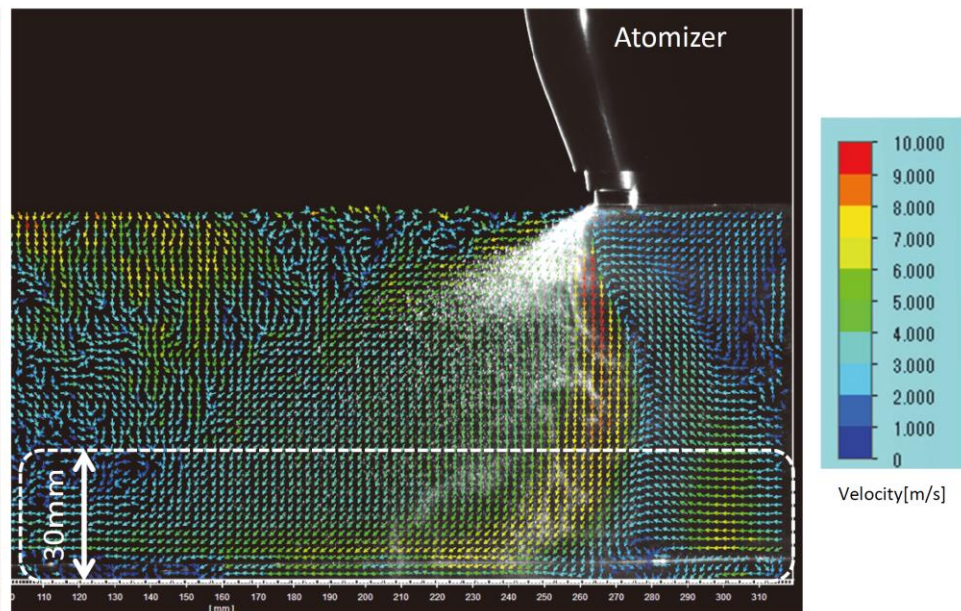
図3-2 高塗着効率塗装機
