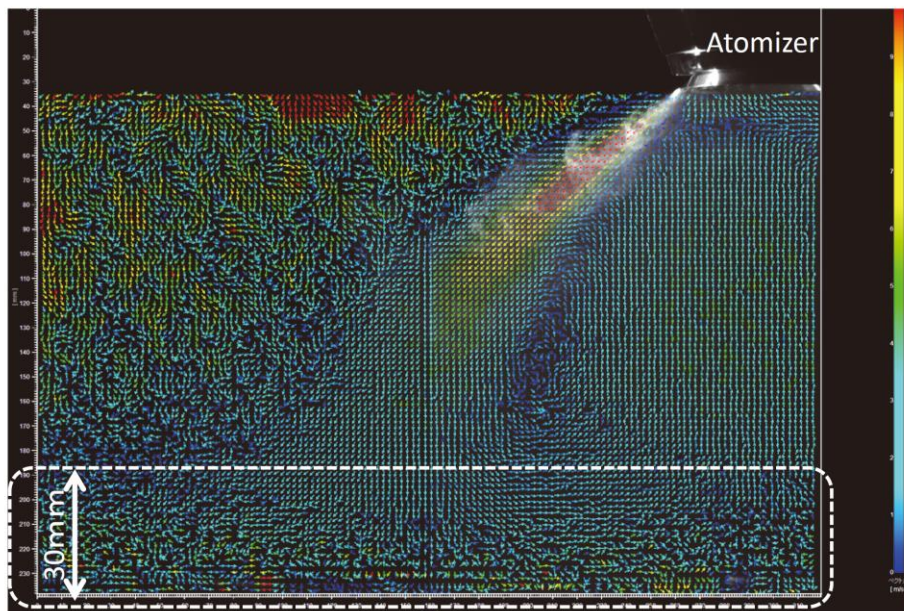
図4-1 従来塗装機
