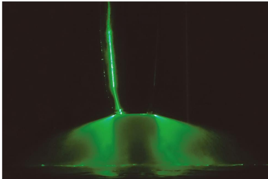
図3-2 高塗着塗装機 塗装距離: 100mm
