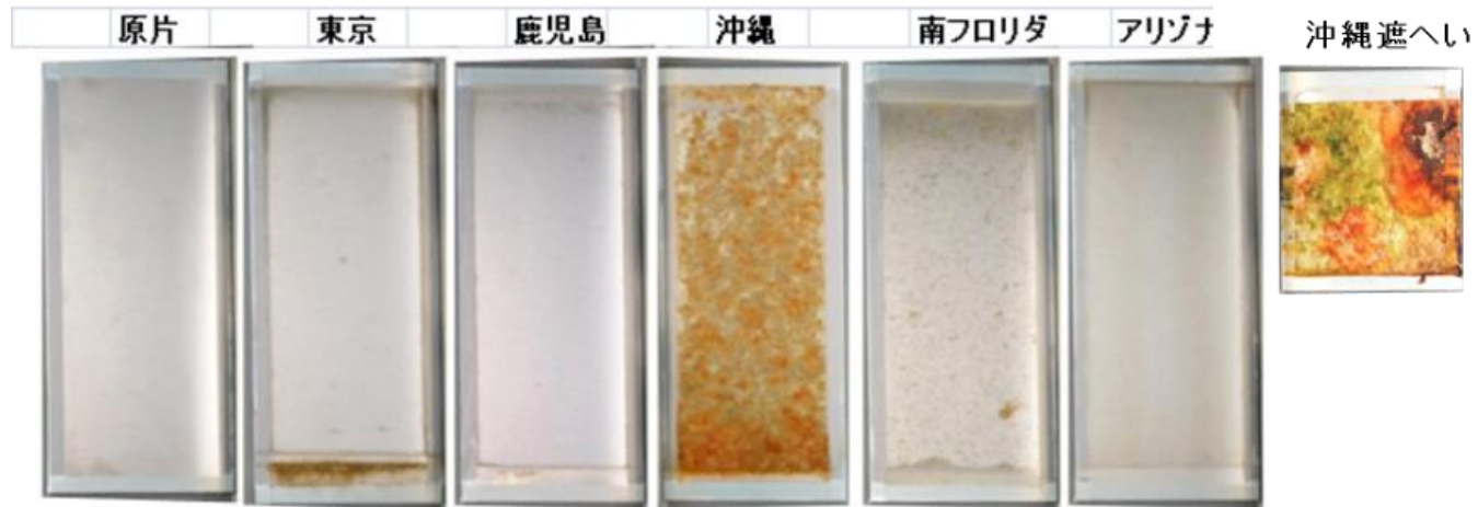
図4 5暴露地におけるSUS430の暴露24ヶ月後
