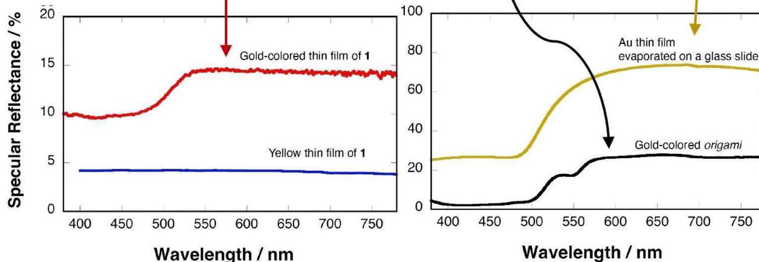
図3 金色多結晶膜と他の金色材料との比較
