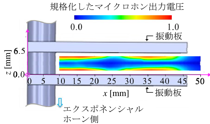
図2 2枚のたわみ振動板間に形成した定在波音場の音圧分布
