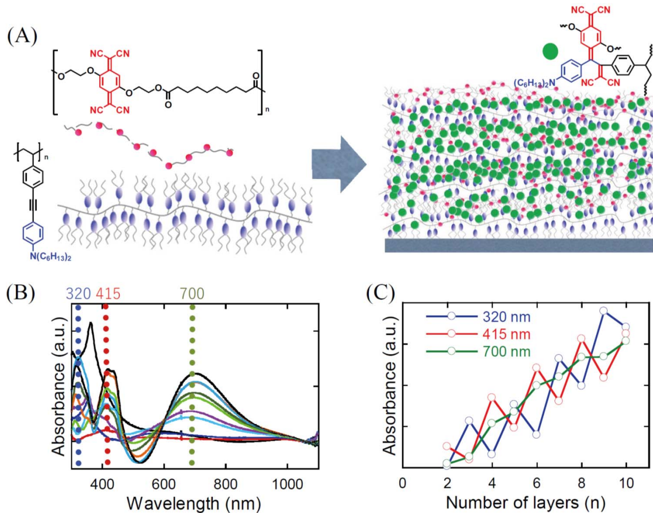
図9 (A) 電子密度が高いアルキンを有するポリスチレン誘導体とTCNQポリエステルとの[2+2]付加環化反応を利用した共有結合型交互積層膜の作製と積層数による (B) 吸収スペクトルおよび (C) 吸光度の変化
