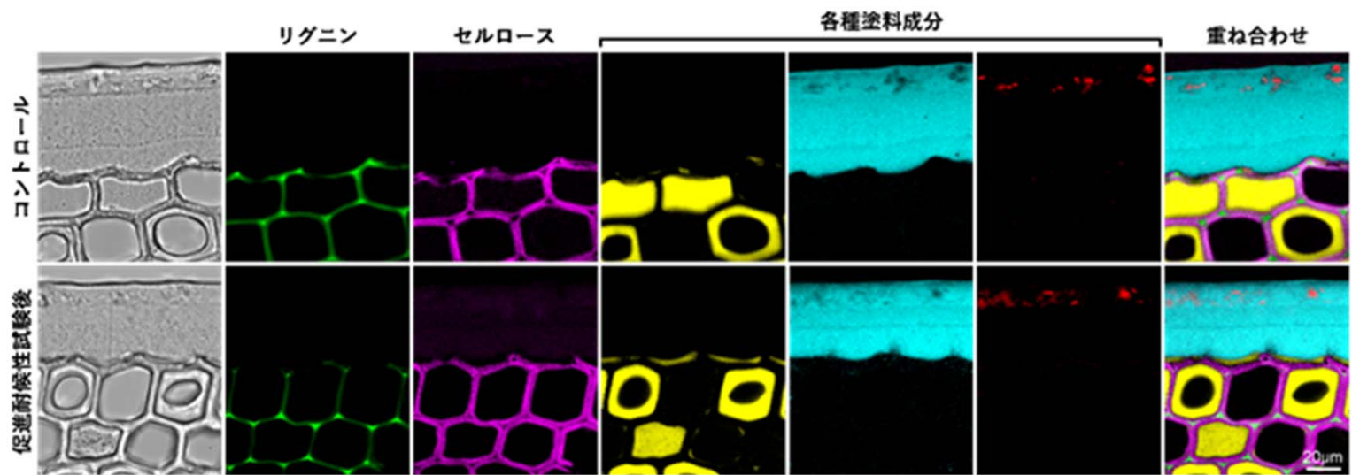
図6 促進耐候性試験前後での塗装木材の表層断面における各種成分の分布イメージ。
