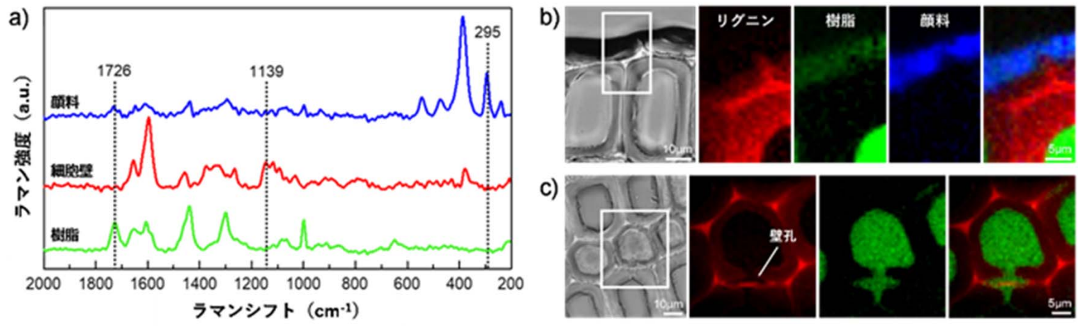
図5 塗装断面におけるラマンマッピング分析 101) 。 a) 細胞壁と塗料成分のラマンスペクトル b) 表層付近の成分イメージ c) 表層から数細胞下方の成分イメージ
